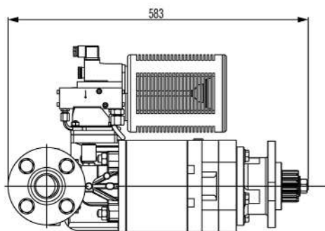
Druckluftanlasser für Motorlinkslauf Compressed air starter for engine counter clockwise rotation 39.5kg
