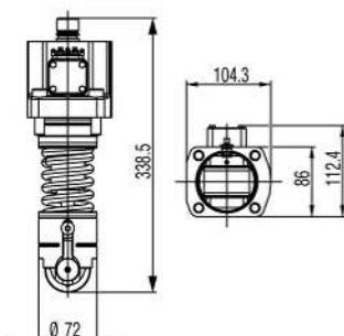
Hochdruckpumpe High pressure pump 9.2kg
