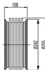
Abgaskompensator (für STC-Leitung) Exhaust gas expansion joint (in STC-pipe) 4.3kg
